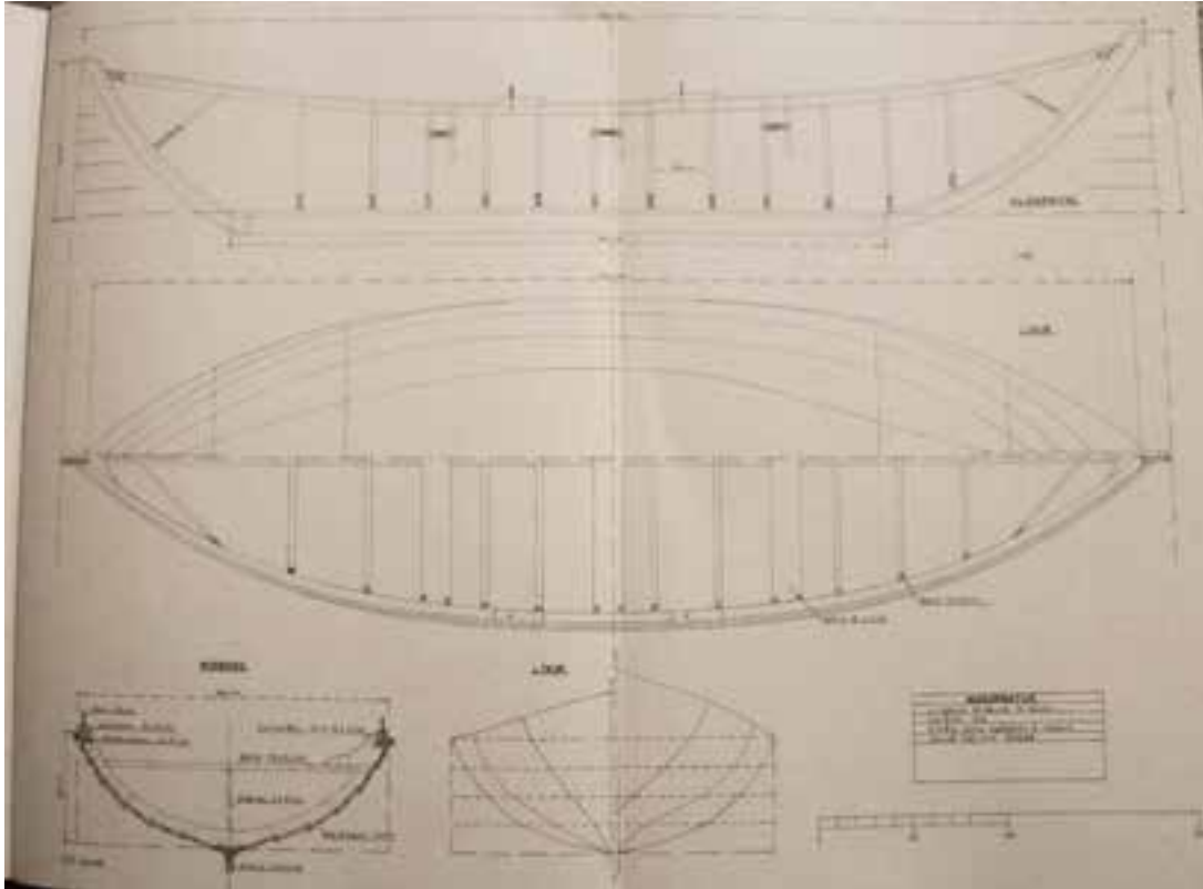
Teikning af Mánárbát, sem sýnir vel lagið á bátum Júlíusar Sigfússonar. Úr Ísl. sjávarhátum I. 16
