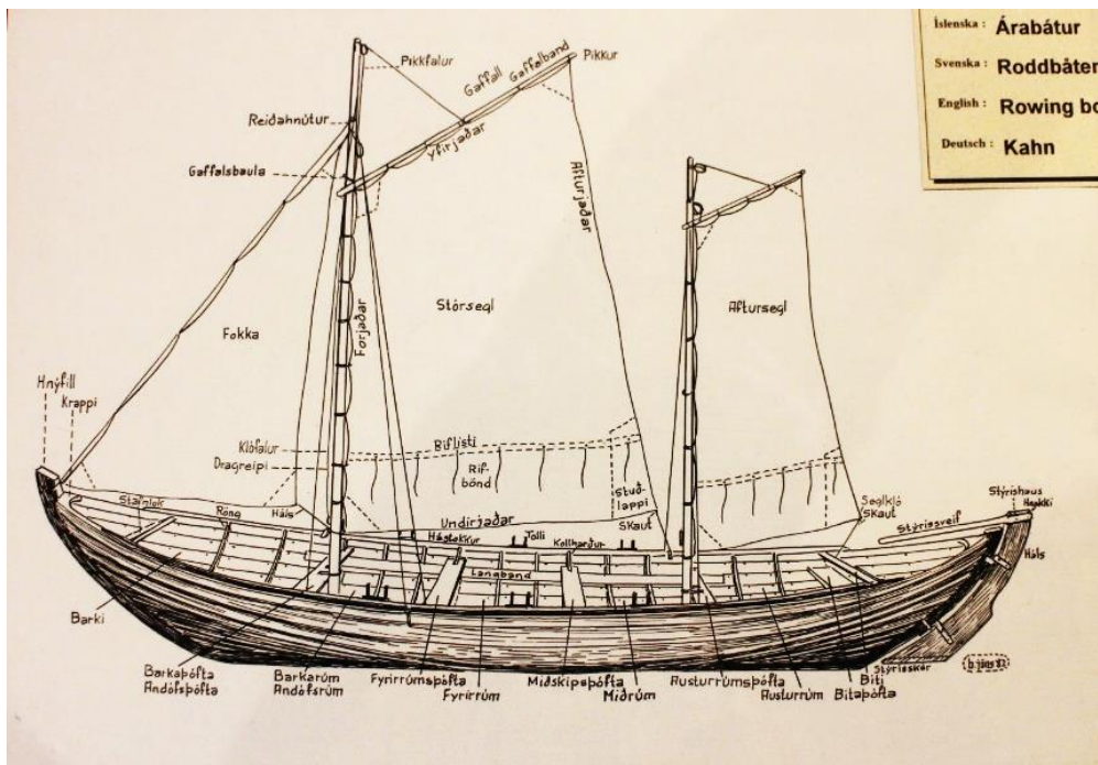
Opinn árabátur. Skýringarteikning eftir Bjarna Jónsson, 1982, með helstu heitum á bátnum og seglabúnaði.
