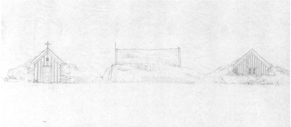
Bænbúsið á Núpsstað, útlit. Teikning arkitektanna Gísla Halldórssonar og Jósefs Reynis.
